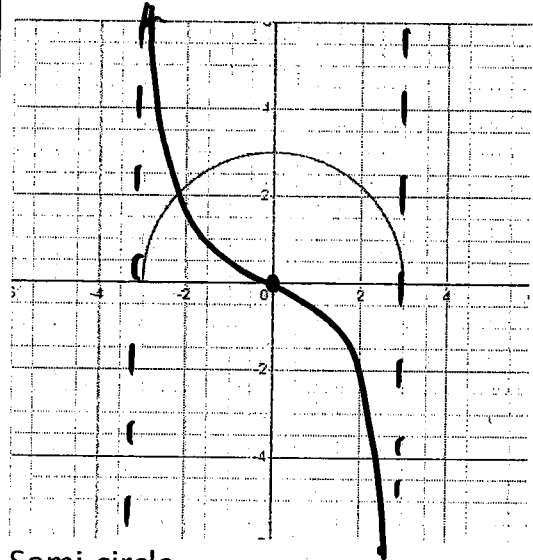
Semi-circle
